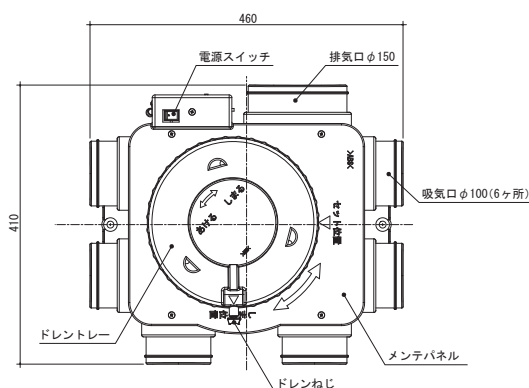
【製品図(ファン)】
