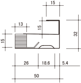
< 製品断面図 >
